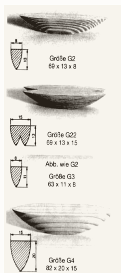
HARZGALLENFLICKE
